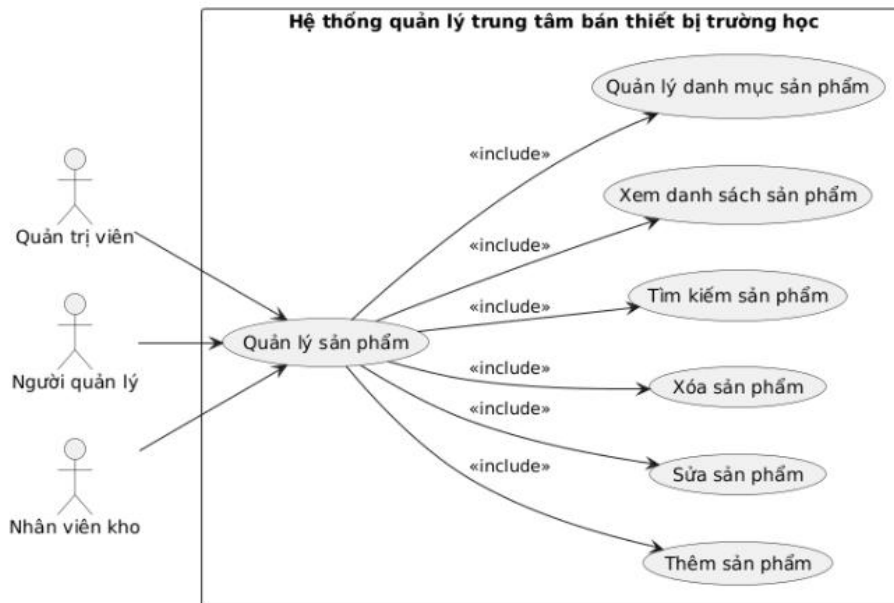
Hình 2.3: Use Case Quản lý sản phẩm
