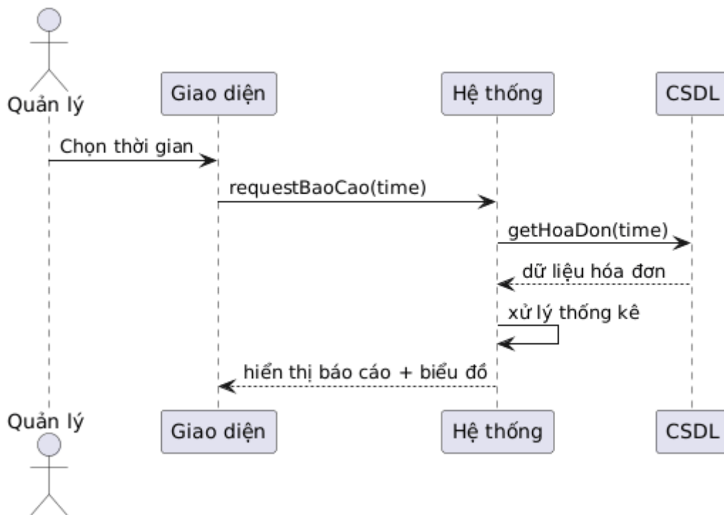
Hình 2.15: Biểu đồ tuần tự xem báo cáo
