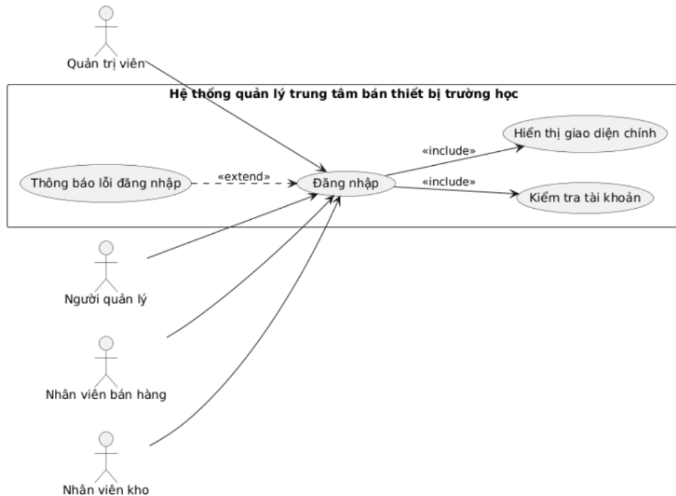
Hình 2.2: Use Case Đăng nhập
