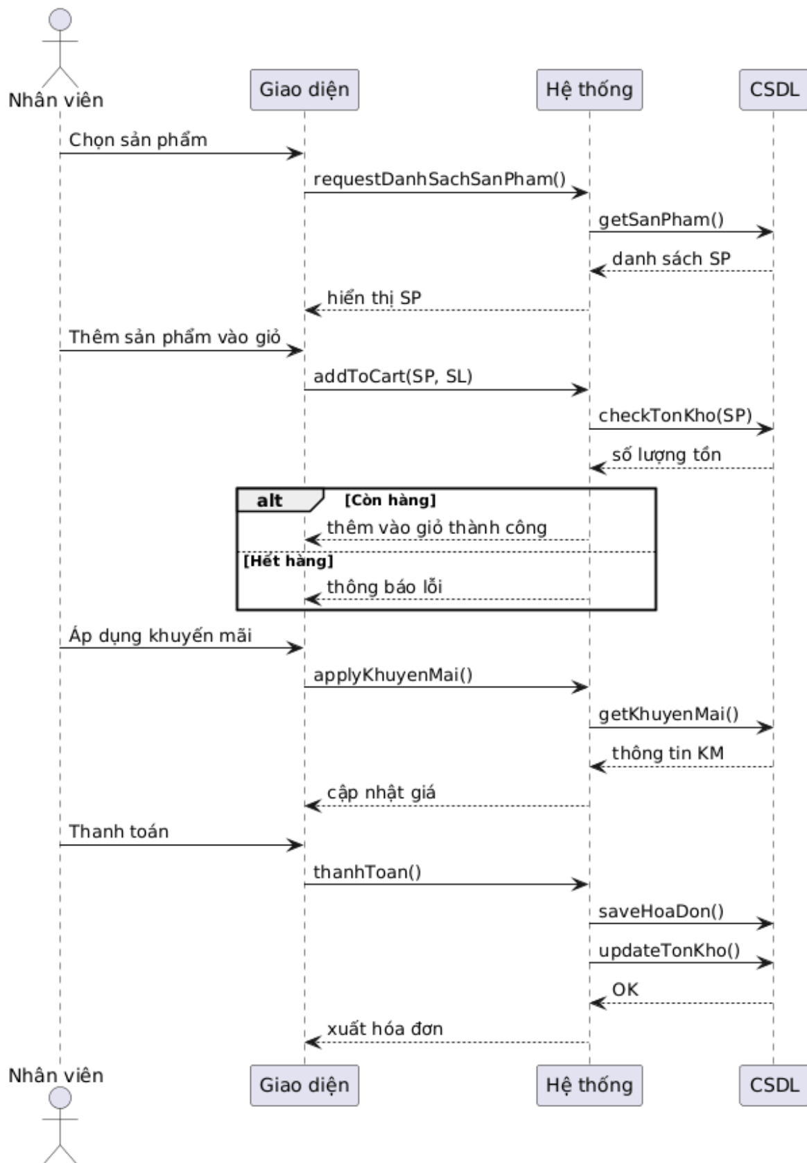
Hình 2.12: Biểu đồ tuần tự bán hàng & lập hóa đơn
