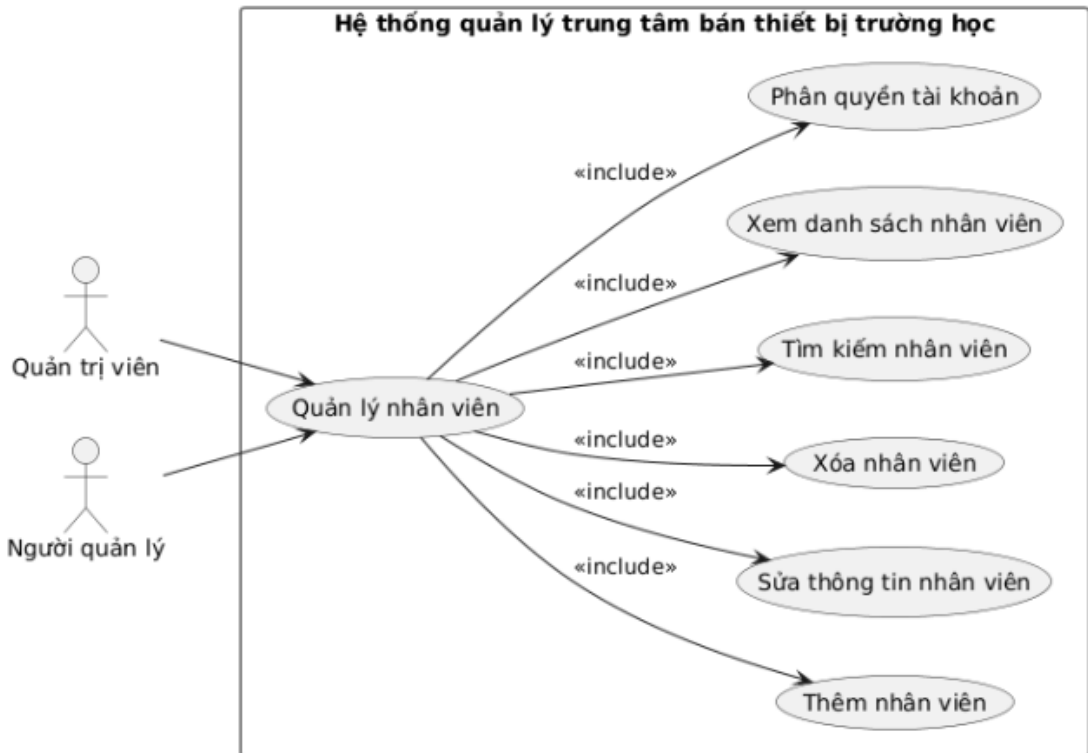
Hình 2.4: Use Case Quản lý nhân viên
