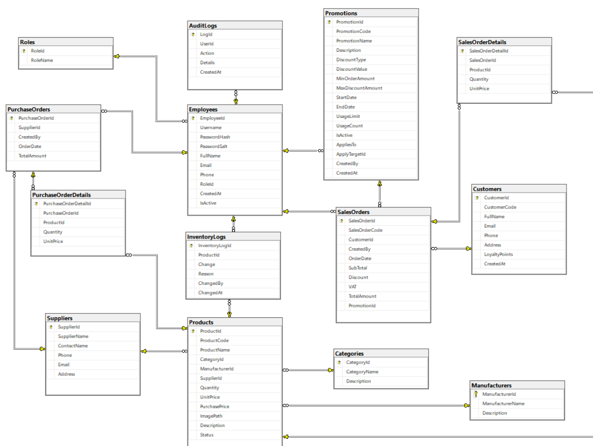
Hình 2.23: Biểu đồ Diagram
