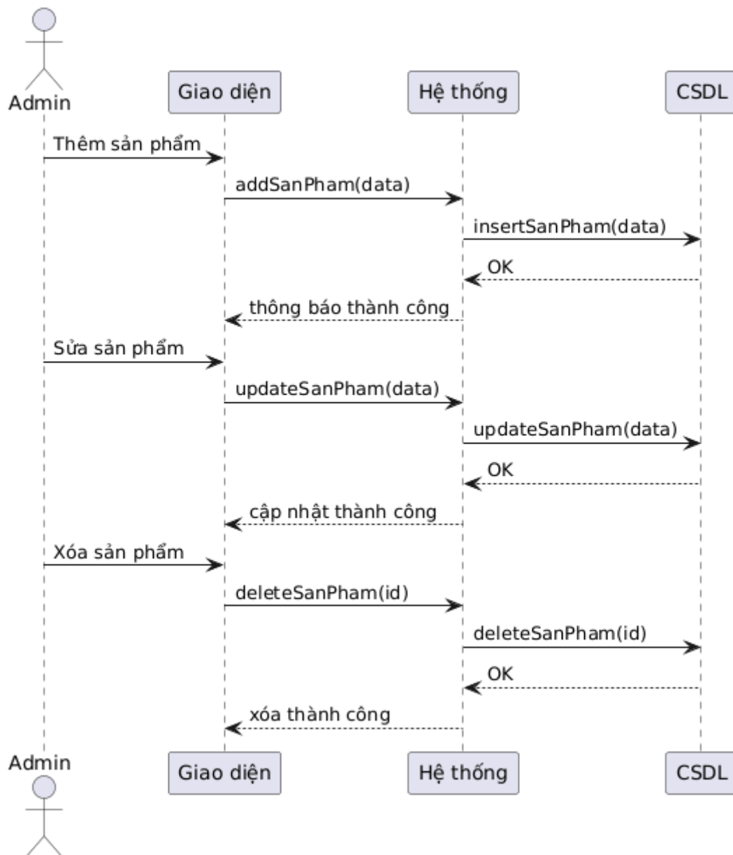
Hình 2.14: Biểu đồ tuần tự quản lý sản phẩm
