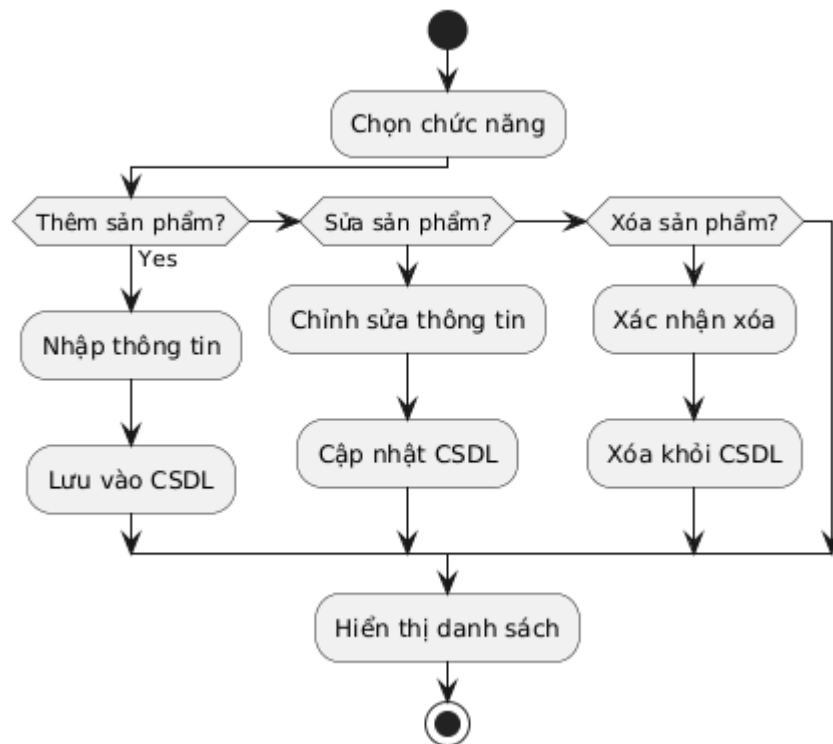
Hình 2.19: Biểu đồ hoạt động quản lý sản phẩm
