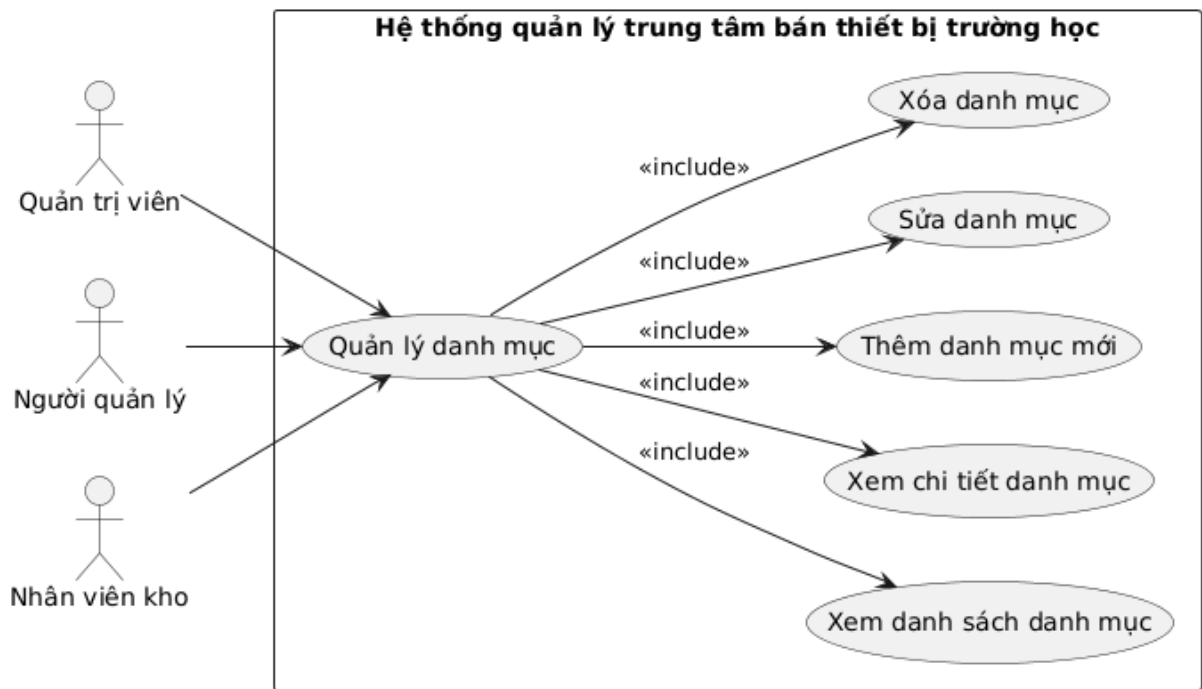
Hình 2.6: Use Case Quản lý danh mục
