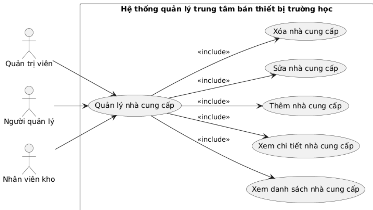
Hình 2.7: Use Case Quản lý nhà cung cấp
