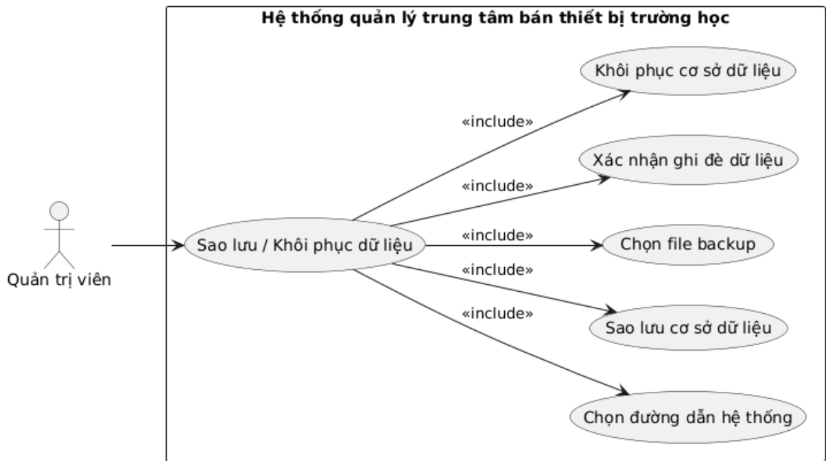
Hình 2.10: Use Case Sao lưu / Khôi phục dữ liệu
