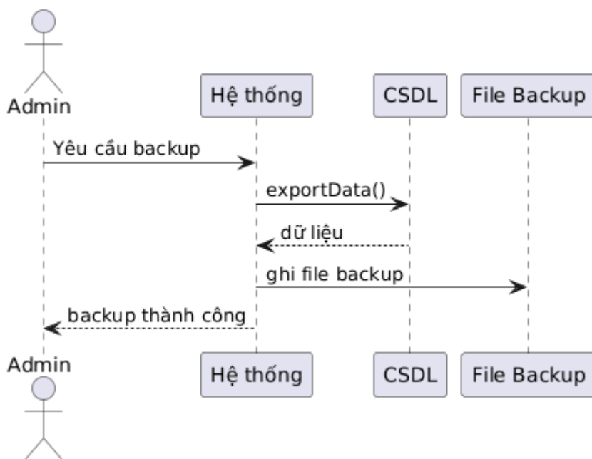
Hình 2.16: Biểu đồ tuần tự backup dữ liệu
