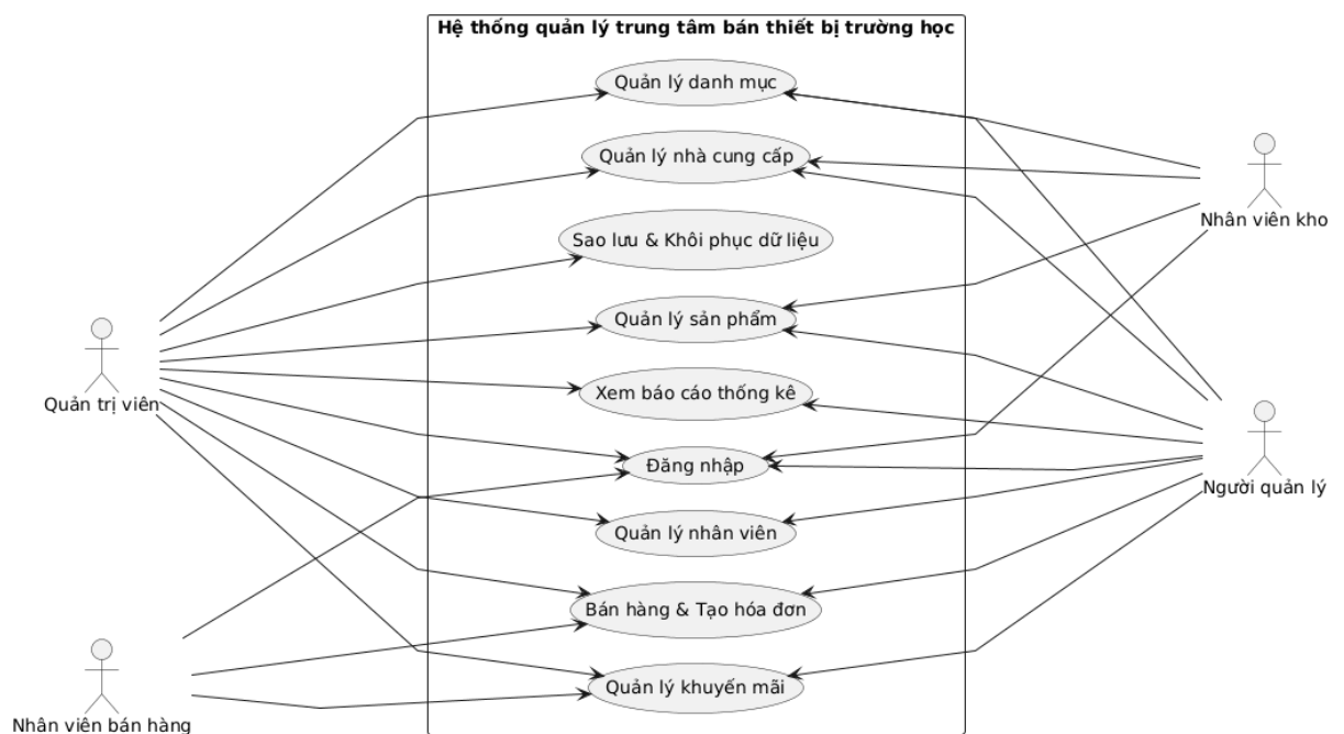
Hình 2.11: Usecase Tổng quát
