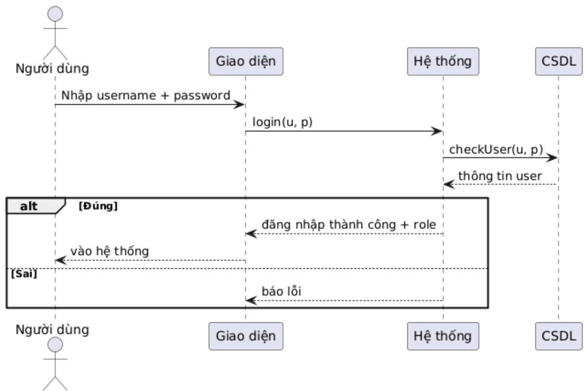
Hình 2.13: Biểu đồ tuần tự đăng nhập & phân quyền
