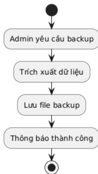
Hình 2.21: Biểu đồ hoạt động backup dữ liệu
