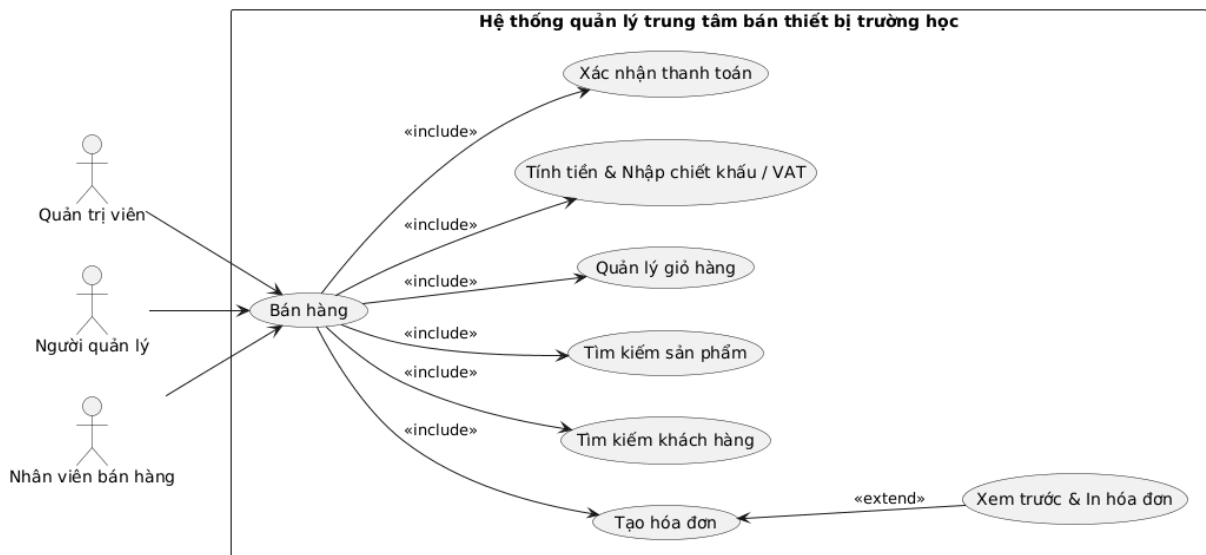
Hình 2.5: Use Case Bán hàng
