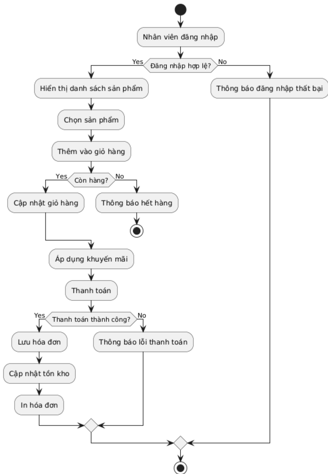
Hình 2.17: Biểu đồ hoạt động quy trình bán hàng
