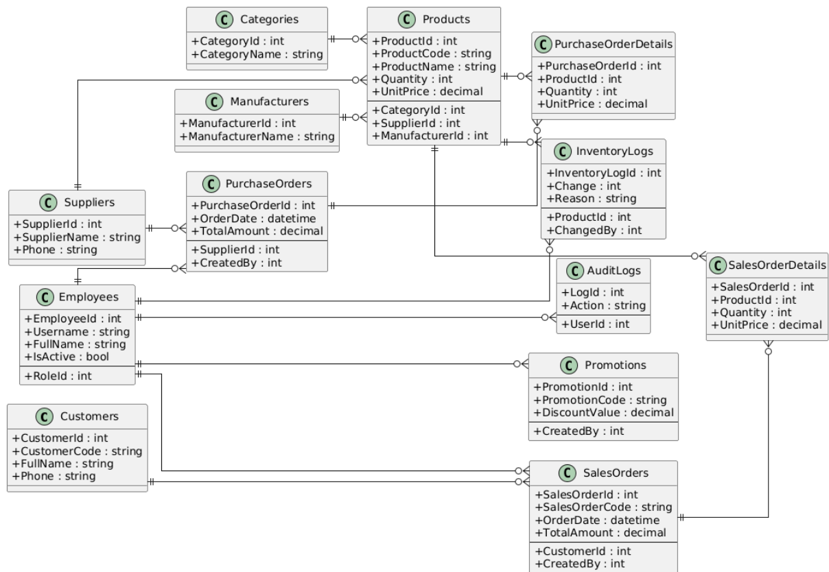
Hình 2.22: Biểu đồ lớp
