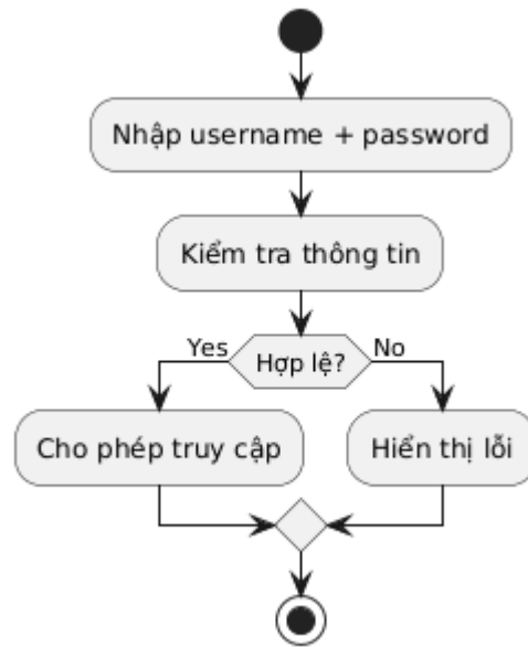
Hình 2.18: Biểu đồ hoạt động đăng nhập
