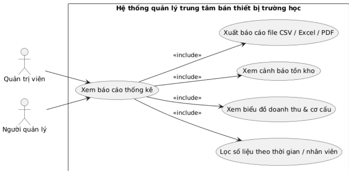
Hình 2.9: Use Case Xem báo cáo thống kê
