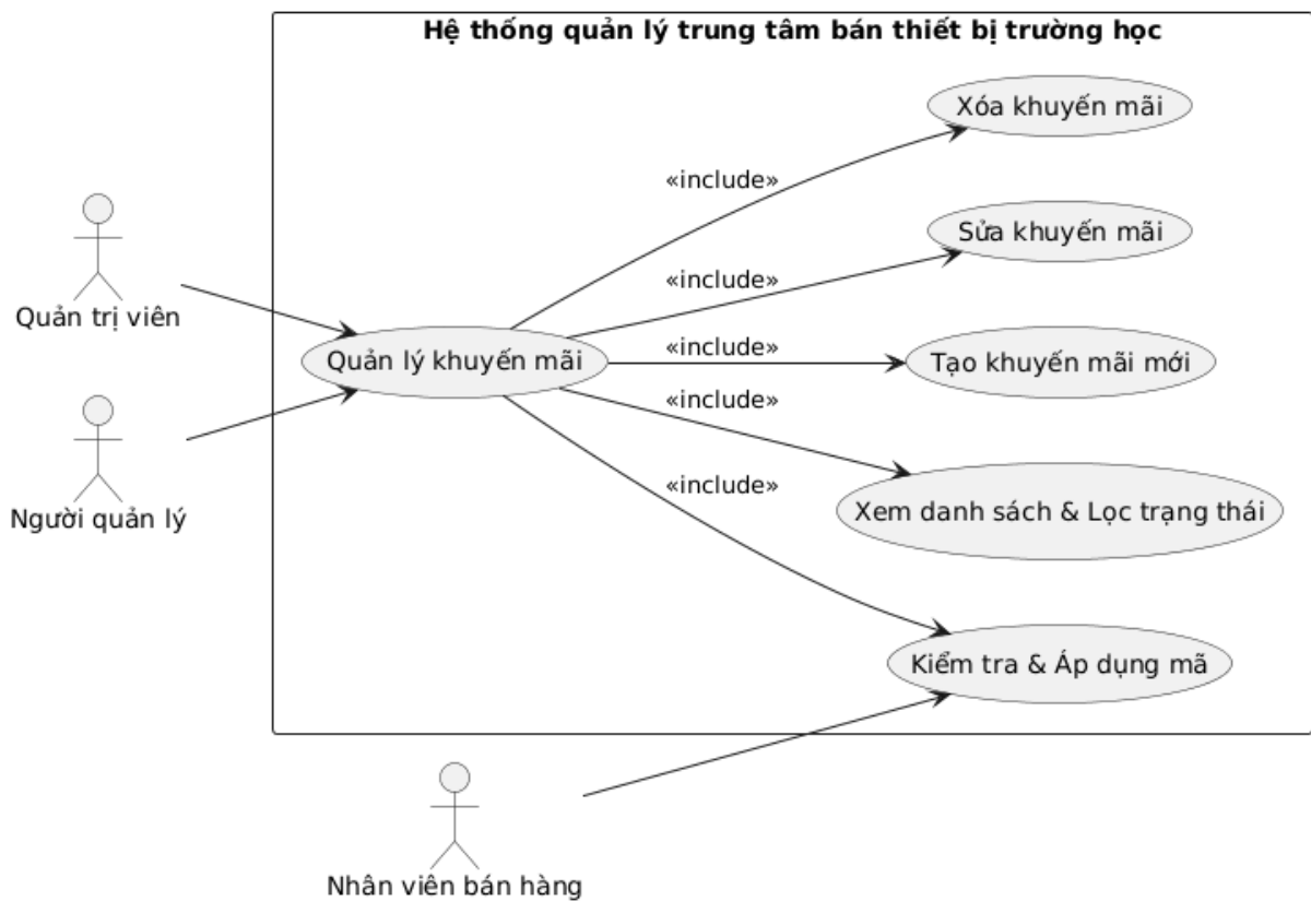
Hình 2.8: Use Case Quản lý khuyến mãi
